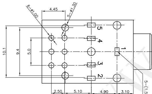
线路板开孔图
